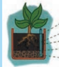
Αυτοποτιζόμενη στεγανή ζαρντινιέρα πήλινη / πλαστική κ.λπ. Υδρομετρητής Χώμα Πορώδες ύφασμα Διογκωμένος άργιλος
